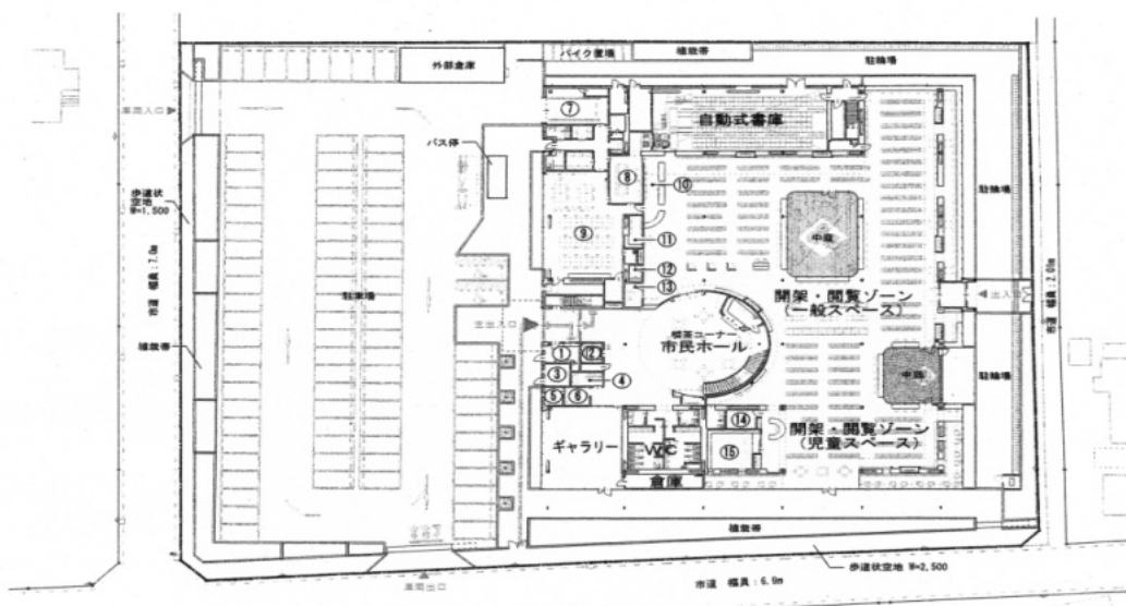
配置図兼1階平面図
